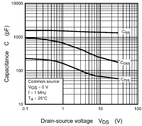
Fig. 8.8 Capacitance - V_{DS}
